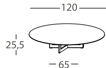
COFFEE TABLE WITH CENTRAL METAL BASE 2,5x5CM / MESAS DE CENTRO CON PIE CENTRAL DE METAL 2,5x5CM / TABLE BASSES AVEC PIED CENTRAL 2,5x5CM
